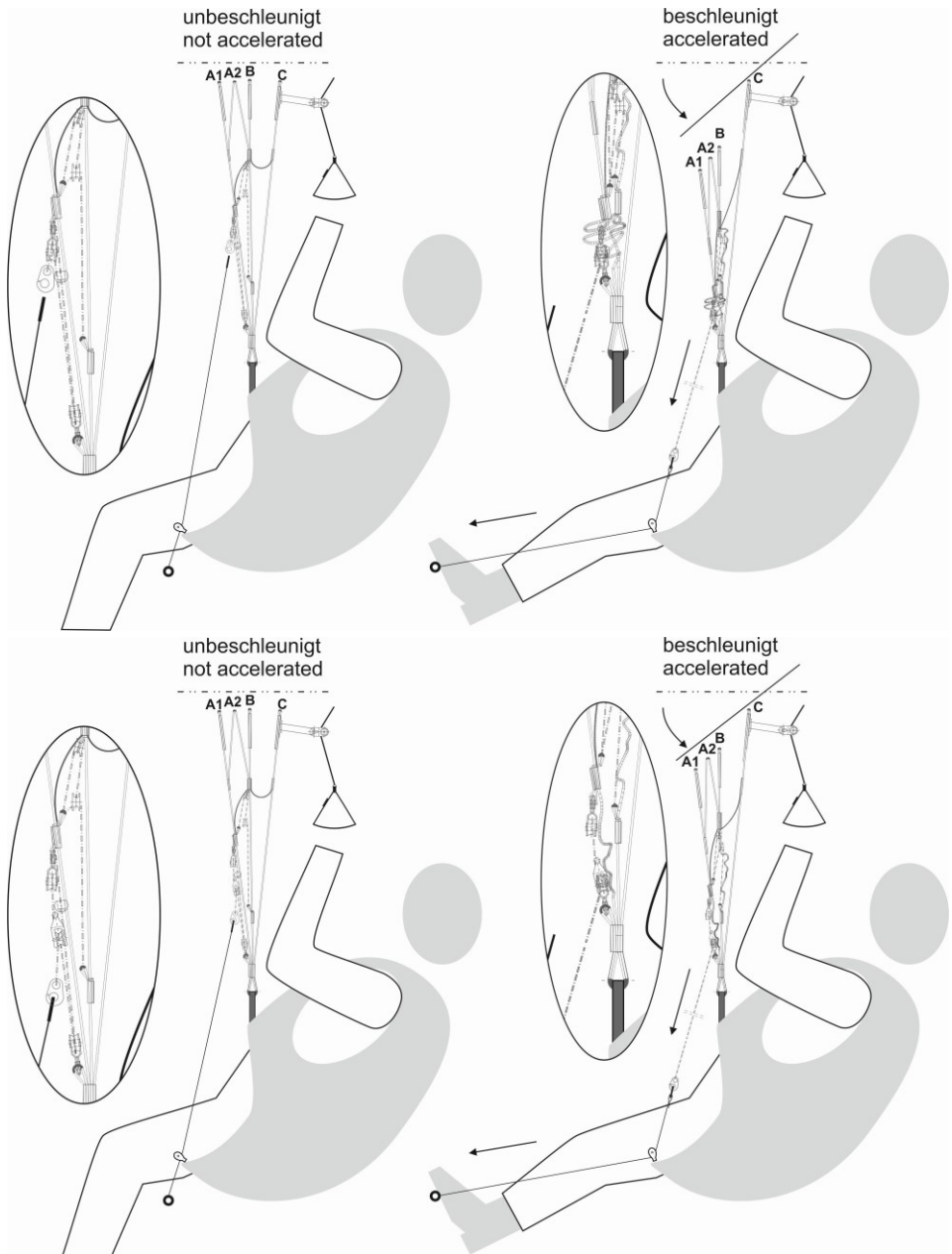
Abb. 8. Funktionsweise Fußbeschleuniger MIURA RS ohne (obere Abbildung) und mit Speedlimiter (untere Abbildung)
