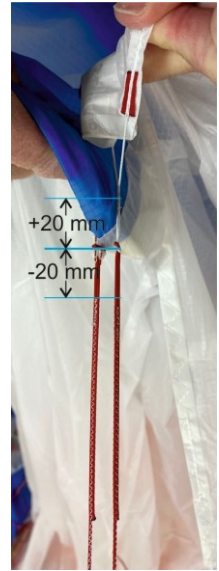
Abb. 14. Maßpunkte für Bremsleinen Schnellcheck
