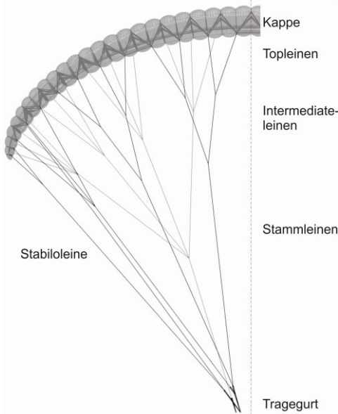
Abb. 1. Gittermodell MIURA RS
