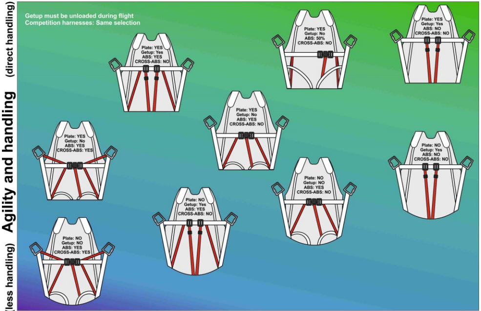
Abb. 12. Übersicht verschiedene Gurtzeuggeometrien und deren Dämpfung
